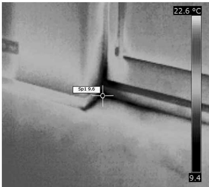
Fotografia przedstawia mostek termiczny progu okna balkonowego – miejsce wykraplania się pary wodnej i potencjalnego rozwoju grzybnii.
