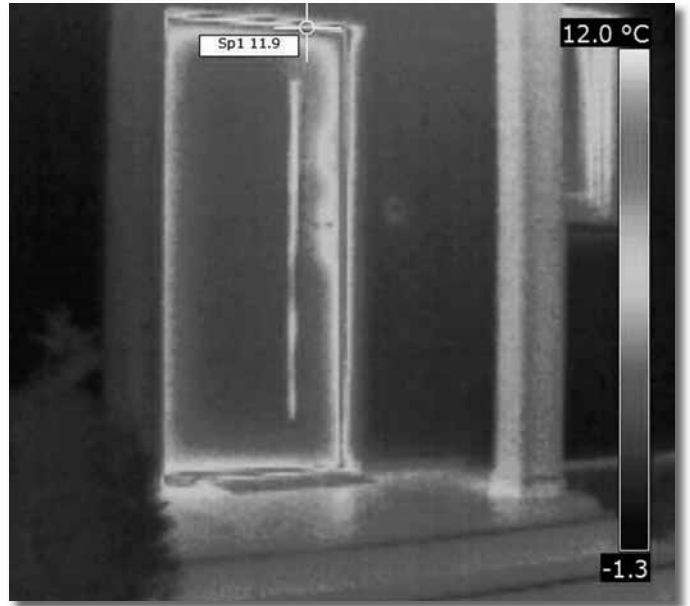
Fotografia przedstawia przykład ucieczki ciepła (mostek termiczny na ościeżnicy drzwi zewnętrznych).
